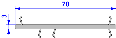
12358 70 mm BAĞ PROFİLİ
