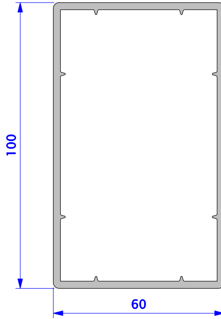
11061 60 x 100 PVC KUTU
