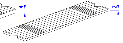
13111 CAM DOLGU 2 mm
