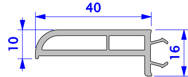
12063 KASA UZATMA 40 mm
